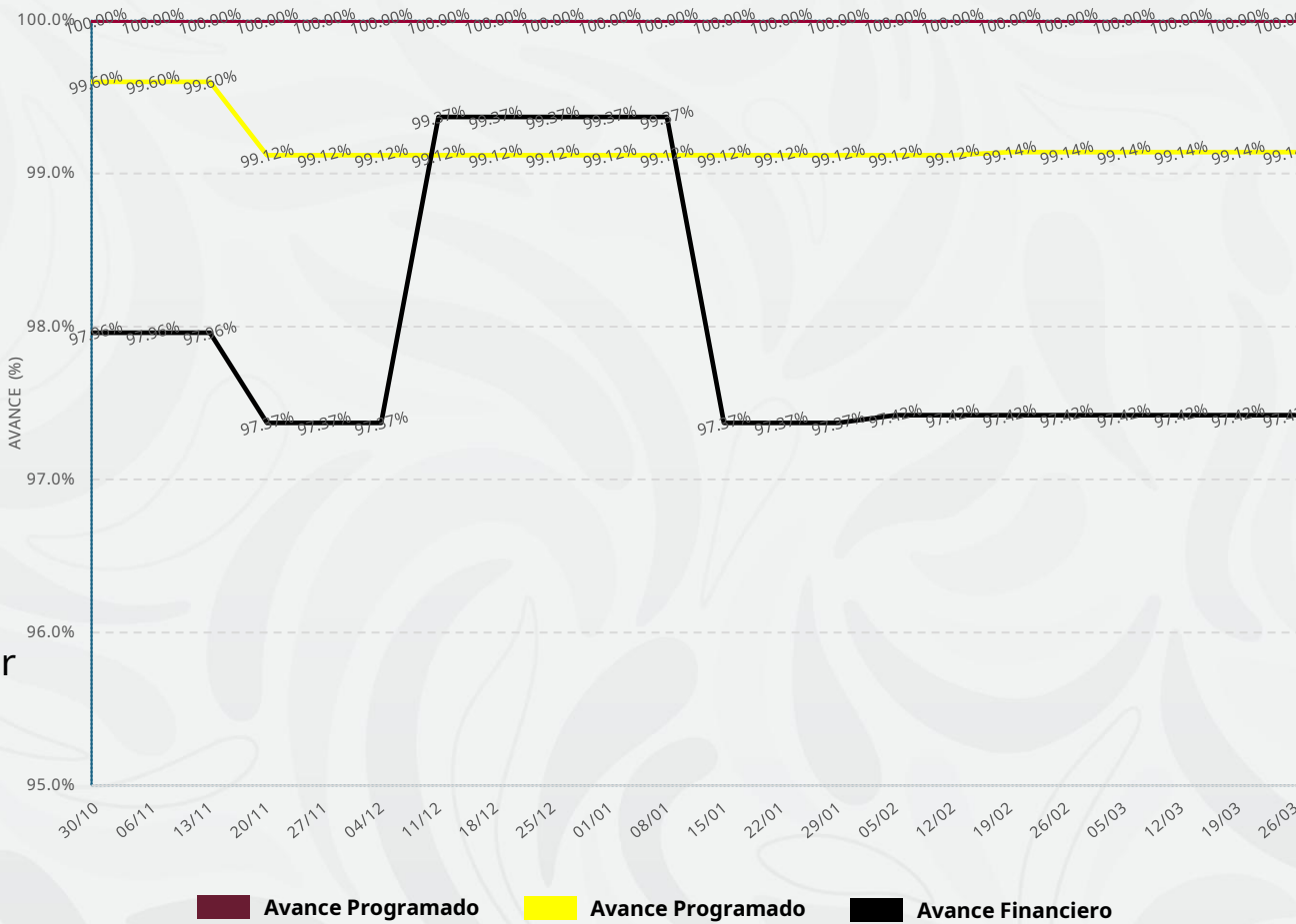
Avance: Programado, Físico y Financiero (%) Mitla - Tehuantepec
